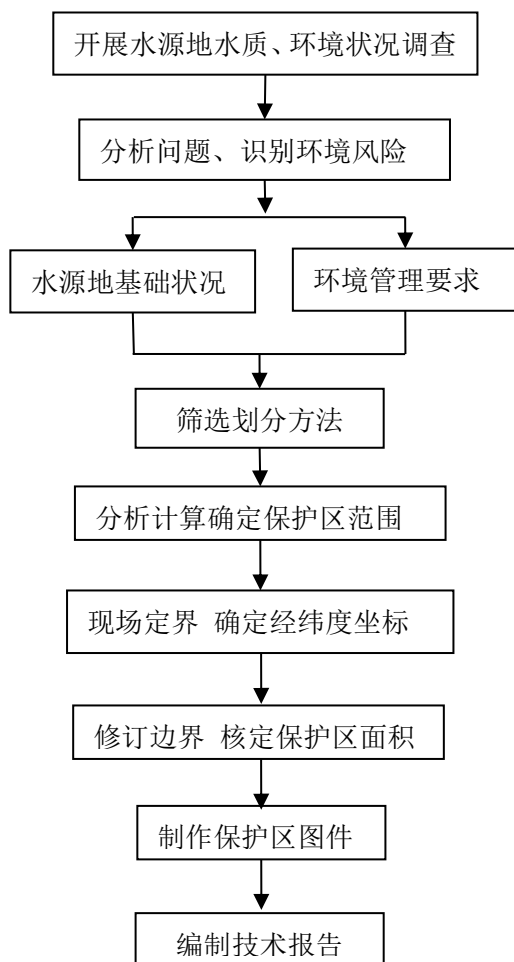
图1 饮用水水源保护区划分技术步骤
